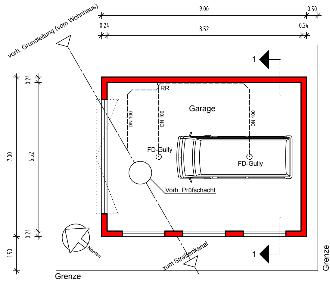
Grundriss
