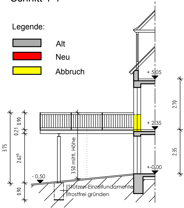
Schnitt 1-1
