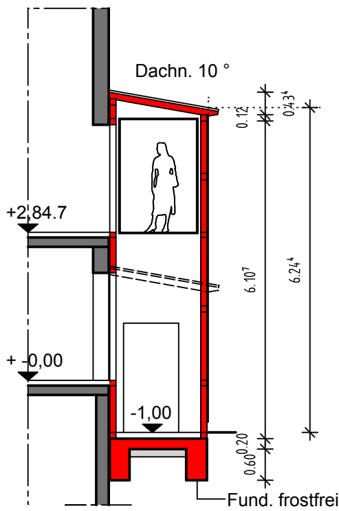
Schnitt 1-1
